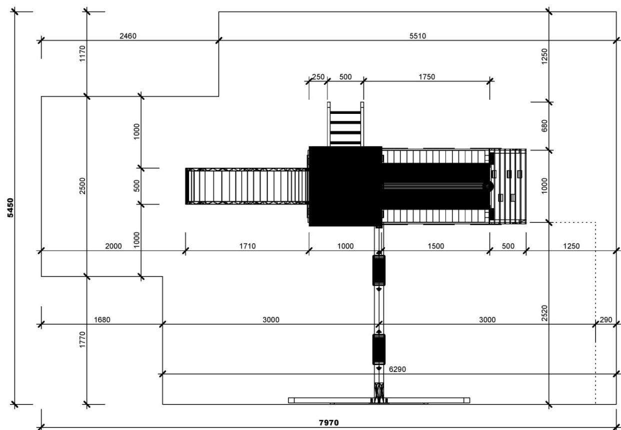
TRAIN - potřebný prostor pro umístění sestavy
