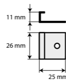
Startovací příchytka terasového prkna k nosníku (P2)
