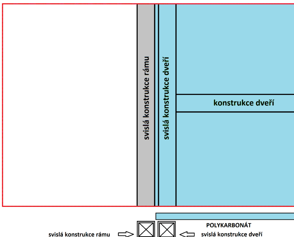
Obr. 8 – plášť dveří ořízněte až podél svislé konstrukce rámu dveří
