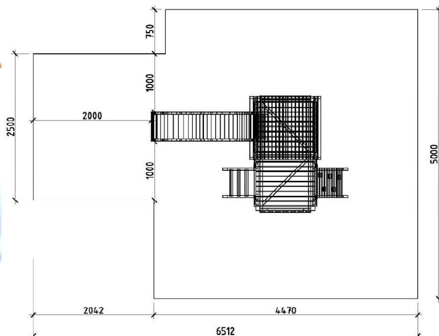
Obr. 2 Dopadová plocha
