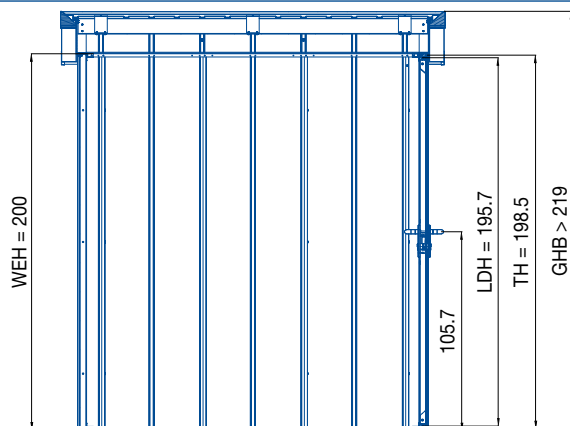
Zahradní domky na nářadí Juno se sedlovou střechou – pohled z boku
