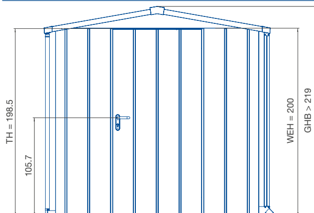
Zahradní domky na nářadí Juno se sedlovou střechou, 1křídle – pohled zepředu
