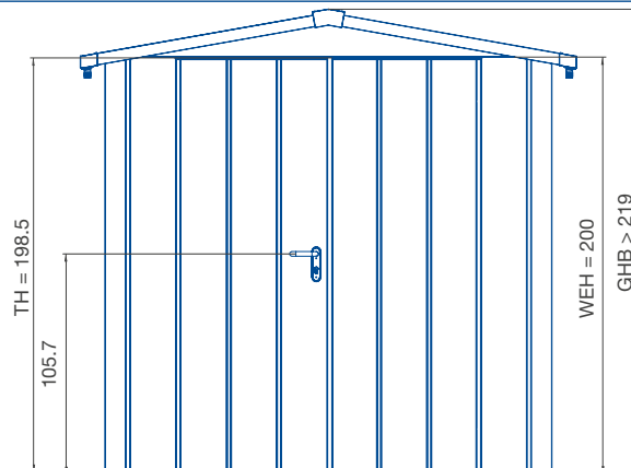
Zahradní domky na nářadí Juno se sedlovou střechou, 2křídle – pohled zepředu
