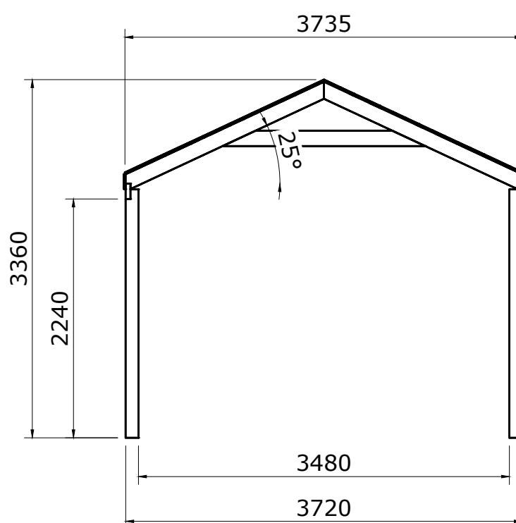
Rechter zijaanzicht
